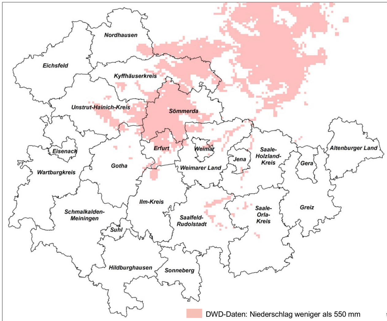
Abbildung: Gebiete < 550 mm Niederschlag im langjährigen Mittel (1991-2019)
